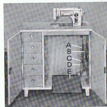
A Gestellrad B Riemen C Riemenaufleger D Zugstange E Trittbrett
