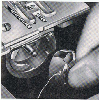
Das Einsetzen der Spulenkapsel
