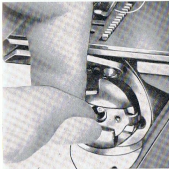
Das Herausnehmen der SpulenkapSEL
