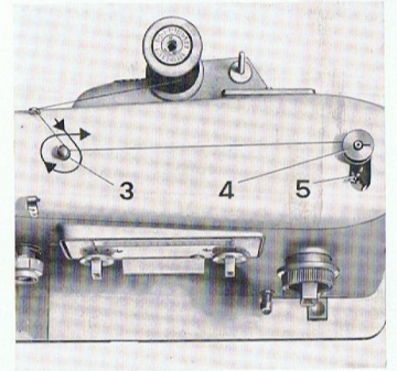
Das Aufspulen des Unterfadens
